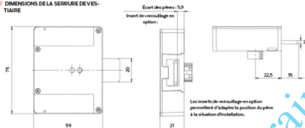
// DIMENSIONS DE LA SERRURE DE VESTIAIRE
